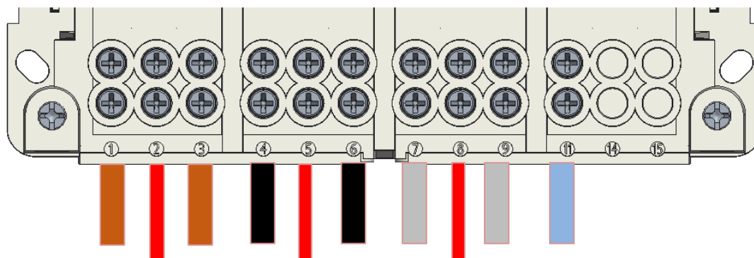
Приклад схеми підключення керуючих входів
