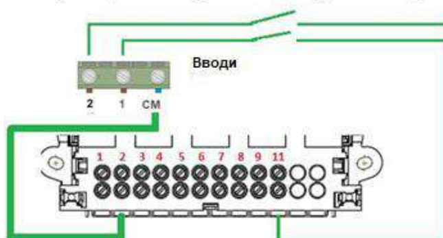
Приклад схеми підключення керуючих входів
